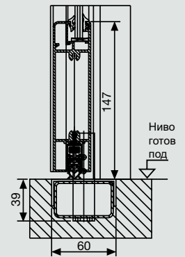
Без долен фалц (за серията, по желание с автоматично спускащо се към пода уплътнение).
