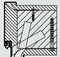
Ограждаща каса Монтаж в зидарията Анкерен дюбел
