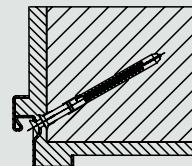
Специална ъглова каса Монтаж с дюбели в основата на жлеба
