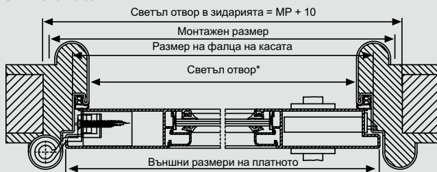
С каса в Roundstyle и Globus-панта
